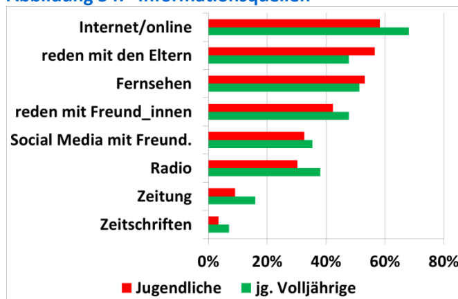
Abbildung 54: Informationsquellen
