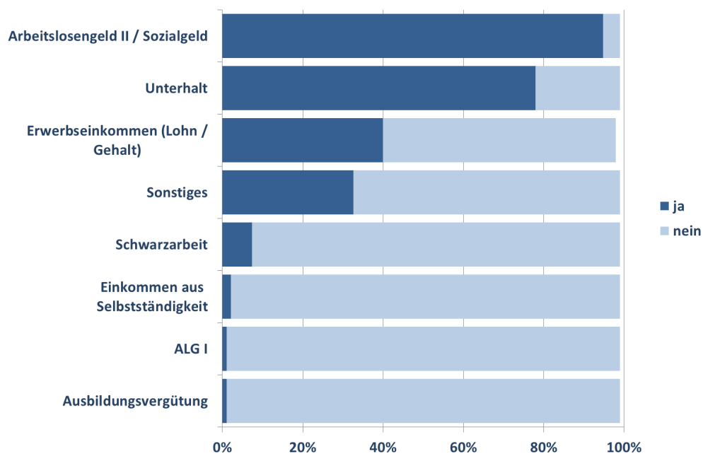
Abbildung 9.1: Einkommensarten
