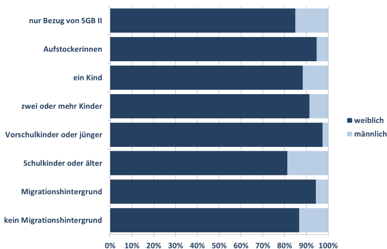
Abbildung 1.2: Subgruppenaufteilung
