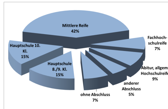
Abbildung 2.1: Allgemeinbildender Schulabschluss
