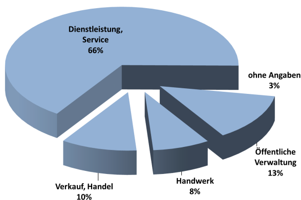
Abbildung 3.10: Hauptarbeitgeber
